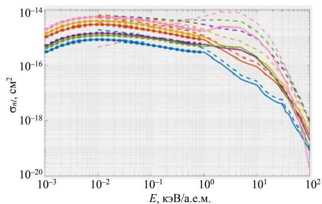
Рис. 10. То же, что на рис. 9, но при перезарядке на атомах водорода в возбуждённом состоянии ( n_H = 2 ): ... — данные [19]; --- — данные [17]; — — комбинация данных [19] и [17], которая использовалась в данной статье
