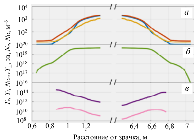
Рис. 5. То же, что на рис. 4, но вдоль линии наблюдения los 2
