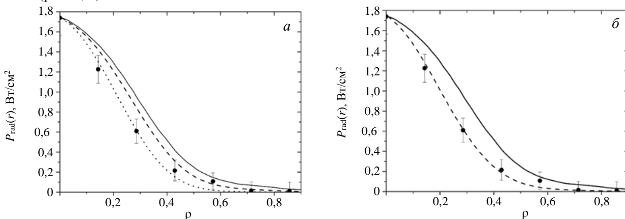
Рис. 6. Сравнение с экспериментальными данными расчётного профиля уточнённой модели с уменьшенным аномальным переносом (● — экспериментальные данные; — — аномальный перенос \times 1 ; - - - — аномальный перенос \times 0,3 ; ... — аномальный перенос \times 0,05 ) (а) и с введённой радиальной токовой зависимостью (● — экспериментальные данные; - - - — с учётом распределения I_{\text{pl}}(r) ; — — без учёта распределения I_{\text{pl}}(r) ) (б)
