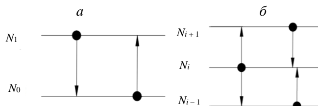
Рис. 2. Процессы, определяющие концентрацию атомов (а) и ионов (б) в корональном балансе
