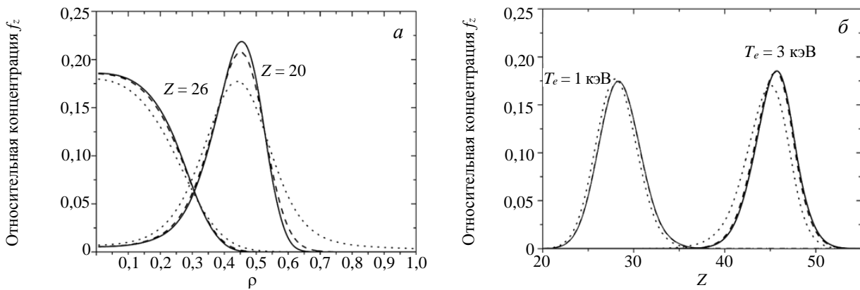
Рис. 3. Профили относительной концентрации ионов с Z = 20 и Z = 26 (а) и распределение по ионным состояниям (б) в корональной модели с обычным и увеличенным в 6 раз переносом: — корона; --- транспорт×1; ··· транспорт×6
