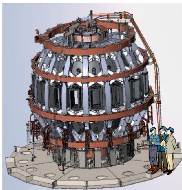
Рис. 7. Модернизируемая установка Т-15. Размеры: R = 1,48 м, a = 0,67 м, поле B = 2 Тл, ток плазмы J \leq 2 МА, вытянутость k \leq 1,9 , мощность нагрева P_{\text{NB}} \leq 6 МВт, P_{\text{EC}} \leq 7 МВт, время удержания энергии \tau_E \leq 0,2 с
