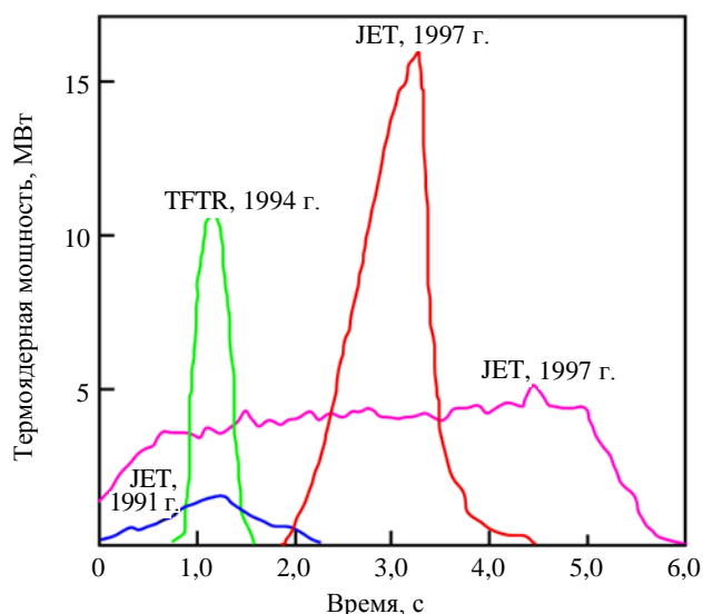
Рис. 5. Термоядерная мощность, генерируемая в D—T-экспериментах на токамаках JET и TFTR
