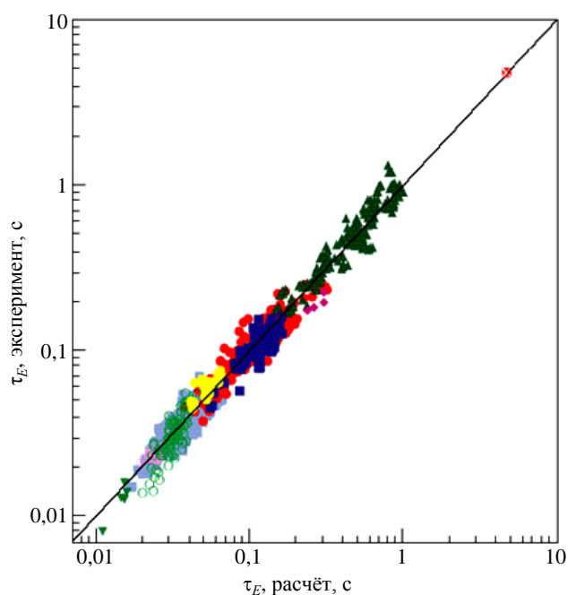
Рис. 6. Сравнение экспериментального энергетического времени жизни с рассчитанным по скейлингу ИТЭР: ■ — ASDEX; ● — DIII-D; ▲ — JET; ◆ — JFT-2M; PBX-M; ○ — PDX; ■ — AUG; ● — C-MOD; ▼ — COMPASS-D; ◆ — JT-60U; * — ITER
