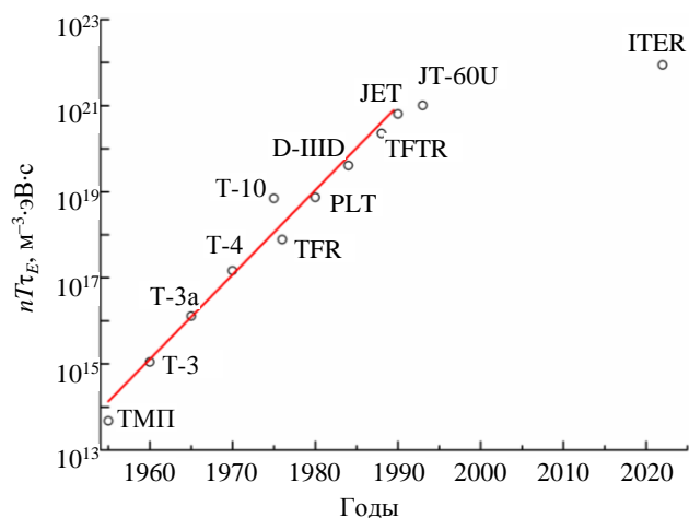
Рис. 4. Наивысшие значения произведения плотности, температуры и времени удержания nT_e\tau_E , полученные на различных токамаках, и планируемое значение параметра nT_e\tau_E для строящейся установки ИТЭР
