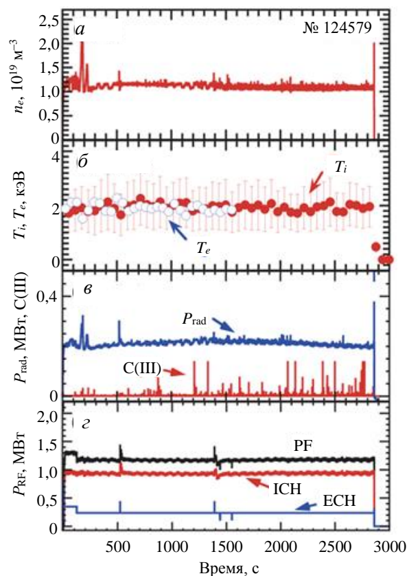
Рис. 9. Импульс длительностью 48 мин на стеллараторе LHD [31]: a — плотность n_e \approx 1,2 \cdot 10^{19} \text{ м}^{-3} ; b — температура T_e \approx T_i \approx 2 кэВ; c — мощность радиационных потерь P_{\text{rad}} \approx 0,2 МВт и свечение линии C(III); d — ИЦ-нагрев 0,9 МВт + ЭЦ-нагрев 0,3 МВт; рабочий газ гелий + 10% водорода
