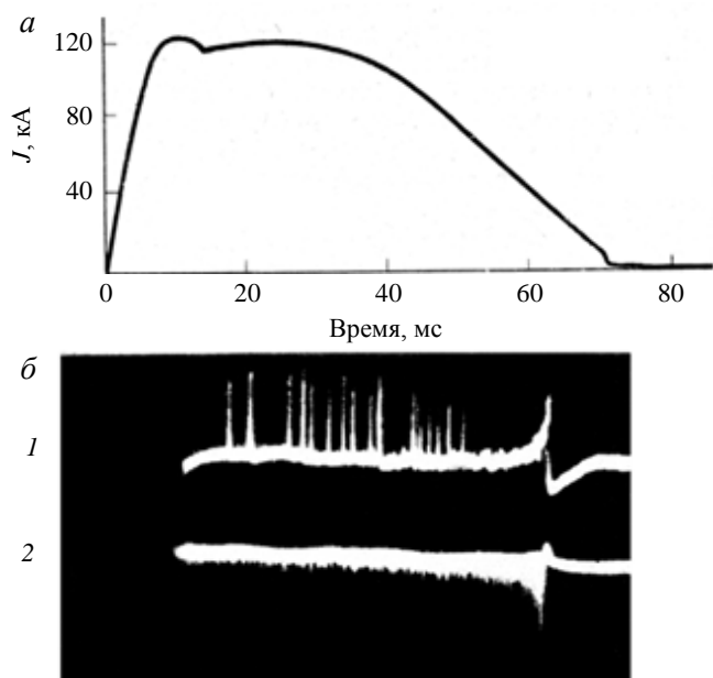
Рис. 2. Один из первых разрядов на токамаке Т-3а, в котором наблюдались нейтроны: а — осциллограмма тока; б — сигнал борного счётчика, регистрирующего нейтроны (1), сигнал сцинтиляционного счётчика, регистрирующего \gamma -излучение (2)
