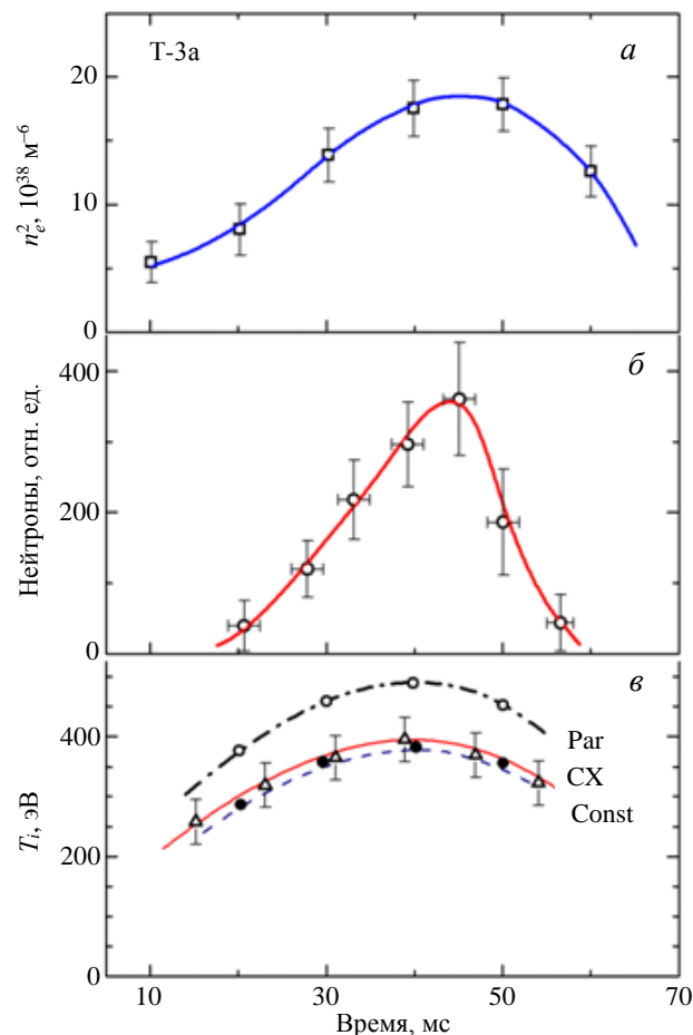
Рис. 3. Изменение квадрата средней плотности плазмы со временем на токамаке Т-3а (а), изменение интенсивности нейтронного излучения (б), ионная температура, определённая по спектрам нейтралов перезарядки (СХ) и по интенсивности нейтронного излучения в предположении однородного (Const) и параболического (Par) распределения температуры и плотности (в)
