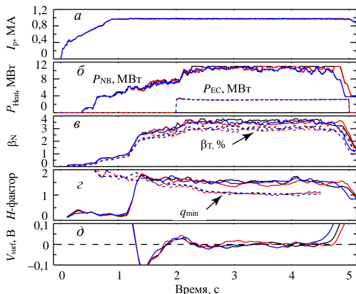
Рис. 8. Безындукционный разряд на токамаке DIII-D: a — ток разряда I_p ; b — мощность нагрева ( P_{\text{Heat}} ) пучком быстрых нейтралов P_{\text{NB}} и СВЧ-волнами P_{\text{EC}} ; c — нормированное давление плазмы \beta ; d — H-фактор и минимальный по сечению запас устойчивости q_{\text{min}} ; e — напряжение обхода V_{\text{surf}} , близкое к нулю
