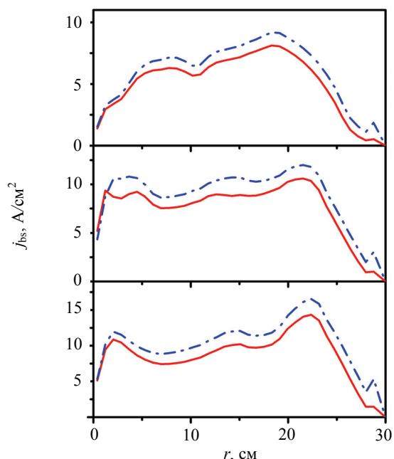
Рис. 11. Профили бутстреп-тока, посчитанные по модели Хинтона-Хазелтайна (—) и Сотера (---): импульс 61 205 (а); импульс 61 208 (б); импульс 61 389 (в)
