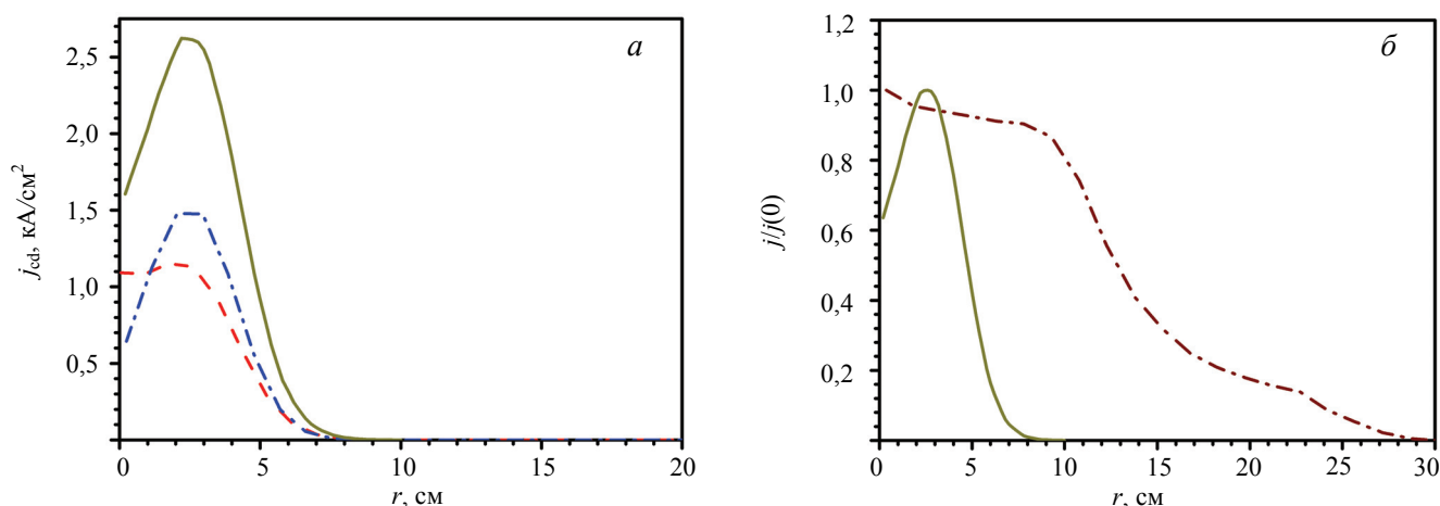
Рис. 13. Импульс 61 389. Плотность ЭЦ-тока: — — — гиротрон 4; - · - · - гиротрон 3; — — — результирующий профиль генерируемого тока (а), нормированные на пиковую величину распределения генерируемого тока (—) и омического тока (- · - · -) (б)
