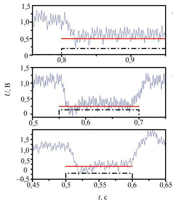
Рис. 12. Экспериментальная осциллограмма напряжения на обходе тора (—), расчётное напряжение на обходе тора (горизонтальная прямая) для импульсов 61 205 (а), 61 208 (б), 61 389 (в): --- — длительность СВЧ-нагрева
