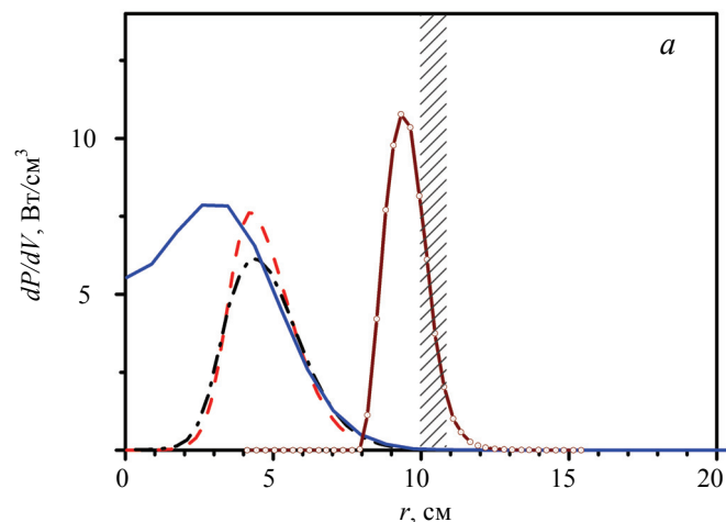
Рис. 8. Профиль плотности поглощённой СВЧ-мощности: — ги́ротрон 4, --- ги́ротрон 1, -.-.- ги́ротрон 2; —○— ги́ротрон 3 (а) и профиль плотности ЭЦ-тока для импульса 61 389 (б)
