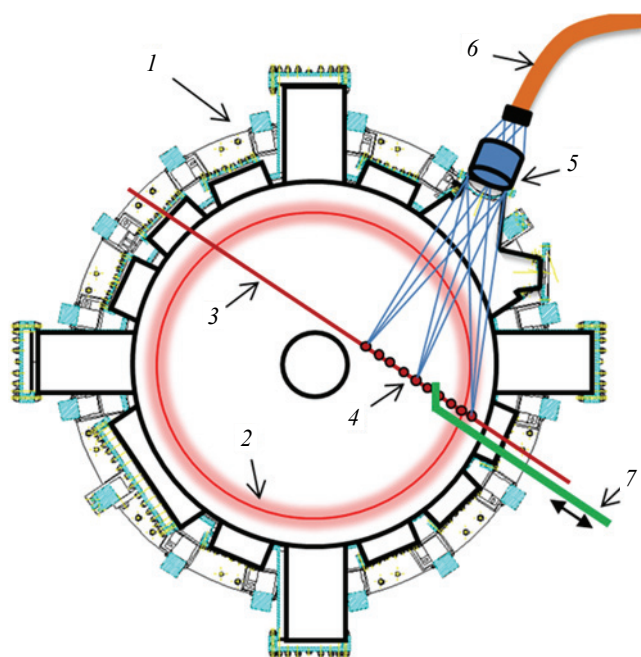
Рис. 1. Размещение дигностики томсоновского рассеяния на токамаке Глобус-М: 1 — сечение камеры в экваториальной плоскости; 2 — внешняя граница плазмы; 3 — зондирующий лазерный пучок; 4 — точки наблюдения; 5 — объектив; 6 — оптоволоконная линия; 7 — система контроля юстировки
