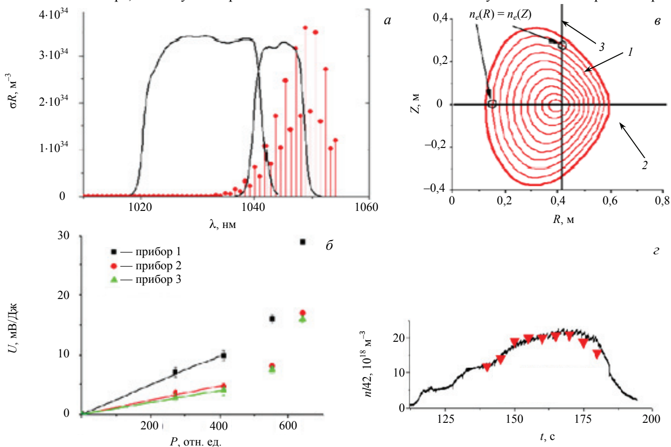
Рис. 3. Сечение рамановского рассеяния лазерного излучения 1055 нм на азоте на фоне первых каналов спектрометра (а); зависимость измеренного значения сигнала рамановского рассеяния от давления газа (б); нормировка на данные интерферометра (в); 1 — магнитная реконструкция равновесной конфигурации по коду EFIT, 2 — проекция лазерной хорды на полоидальное сечение плазменного шнура, 3 — хорда наблюдения интерферометра; временная эволюция концентрации электронов в разряде токамака (з): — — данные интерферометра, \blacktriangledown — данные ТР
