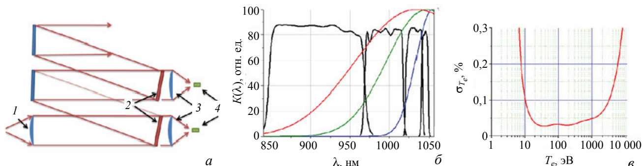
Рис. 2. Принципиальная схема фильтрового спектрометра ( a ): 1 — входной объектив, 2 — спектральный фильтр, 3 — объектив, 4 — приёмник; b — спектральные характеристики каналов спектрометра и наложенные спектры томсоновского рассеяния; c — кривая ошибок измерения температуры для выбранного набора спектральных каналов полихроматора
