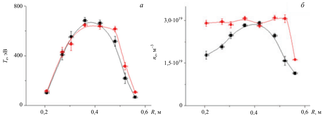
Рис. 5. Распределение температуры (а) и концентрации электронов (б) вдоль большого радиуса плазменного шнура, измеренное в одном разряде до и после L—H-перехода, № 26167: ■ — L-мода; ● — H-мода
