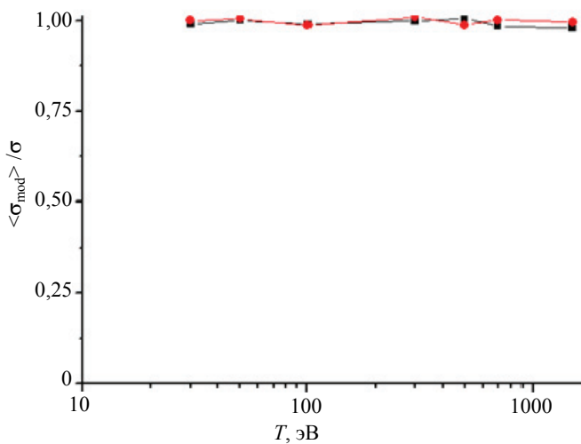
Рис. 4. Зависимость отношений дисперсий распределений температуры и концентрации, полученных путём численного расчёта, к значениям среднеквадратичных отклонений, рассчитанных по формулам для линеаризованного МНК, от температуры: ■ — T_e ; ● — n_e
