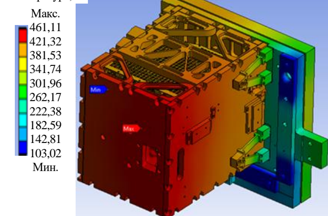
Рис. 7. Профиль температурного распределения в УВЗ СВЛ-диагностики
