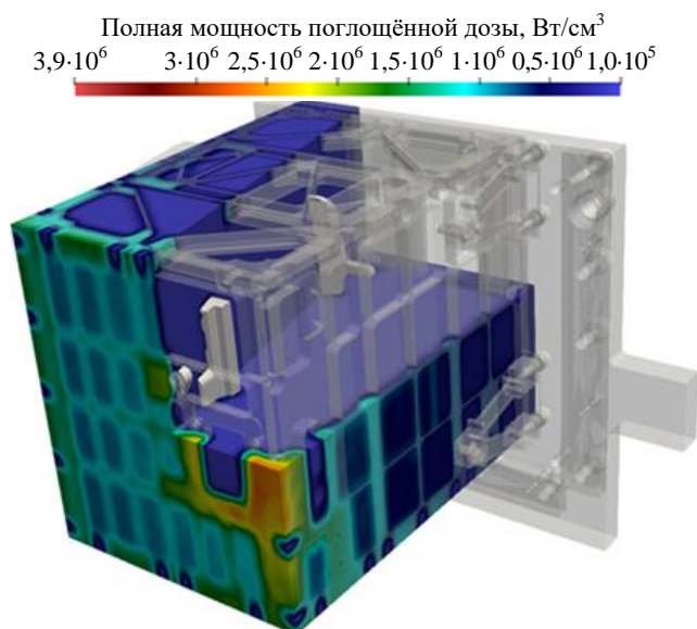
Рис. 6. Профиль полной мощности поглощённой дозы в УВЗ СВЛ-диагностики
