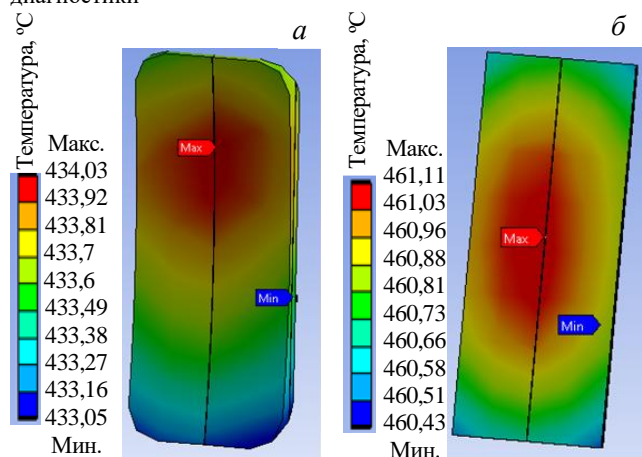
Рис. 8. Профиль температурного распределения в зеркалах M1 (а) и M2 (б) СВЛ-диагностики
