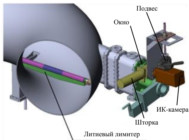
Рис. 9. Схема расположения ИК-диагностики
