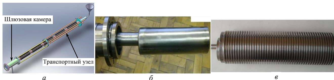
Рис. 2. Криогенная мишень токамака Т-11М: общий вид (а), приёмный элемент (б, в)
