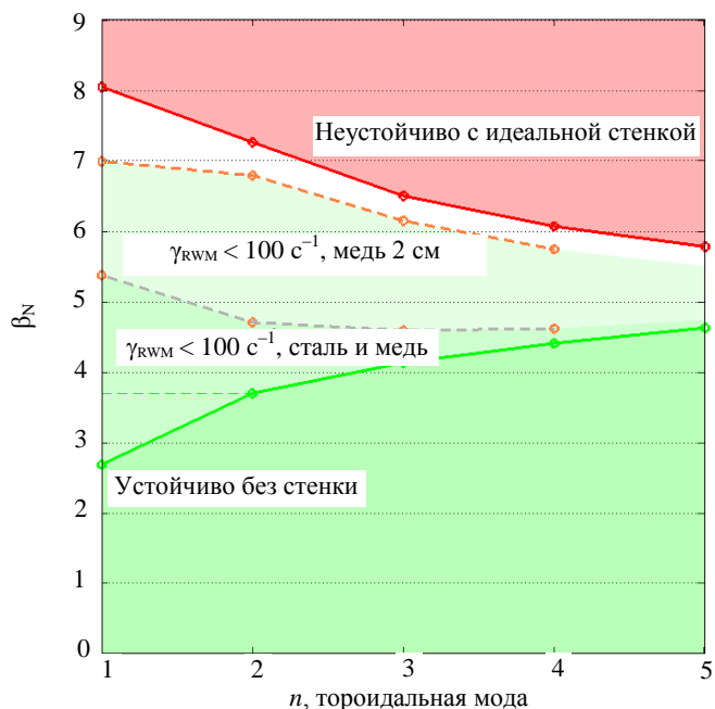
Рис. 5. Предельные значения \beta_N без учёта и с учётом стабилизации проводящей стенкой для внешних винтовых мод n = 1-5 , скинированный ток, I_N = 3
